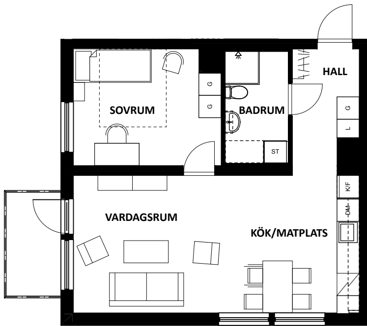
2 RoK 53,5 kvm, V 1:100 20 ST
