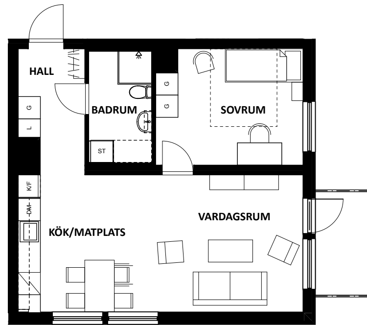
2 RoK 53,5 kvm, H 1:100 5 ST
