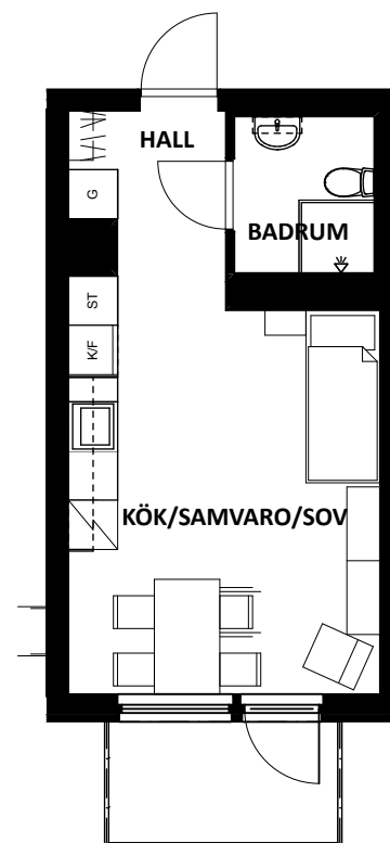
1 RoK 25,5 kvm 1:100 4 ST
