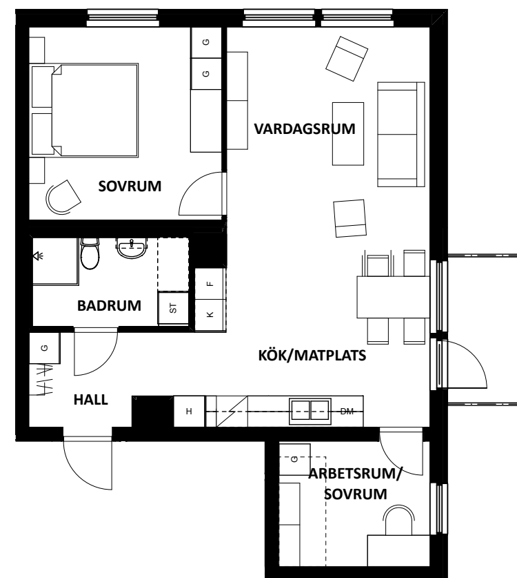
3 RoK 65,8 kvm, H 1:100 4 ST
